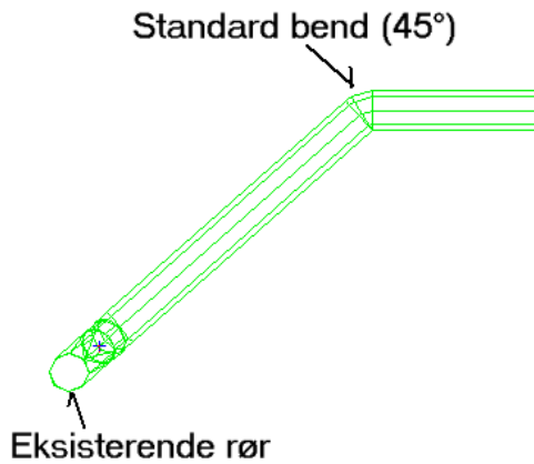
Tilknytning med standard bend. DDS-CAD justerer siste punkt før tilknytning.
