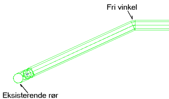
Fri vinkel. DDS-CAD bruker siste punkt før tilknytning, og regner ut vinkelen på bendet, som i de fleste tilfeller vil avvike fra standard grader.
