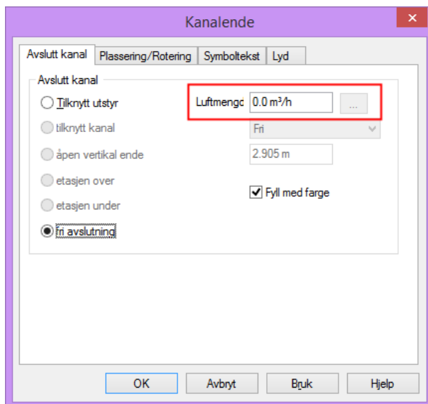
Egenskaper for kanal som er avsluttet med ventil
